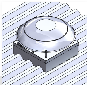
2. Colocar Roof curb o base (provisto por el cliente) y montar el ventilador.
